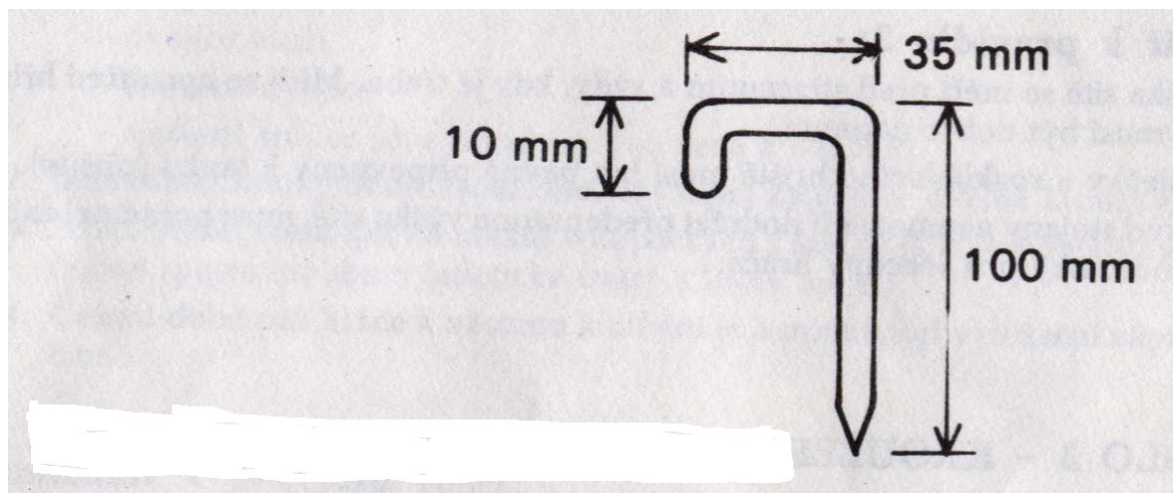
Obr.2 doporučený tvar a rozměry vypínacích kolíků
